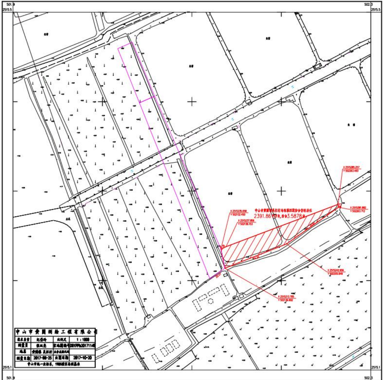
标的 4 图纸
