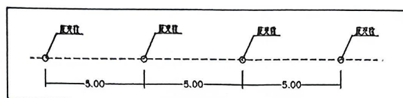
反光柱设置单元平面图示意图
